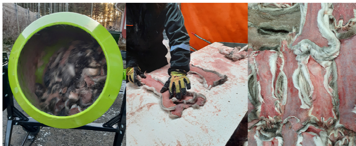
Kuva 4. PoSiHIILI-hankkeessa kehitetty suolausrumpu koipinahkojen suolaukseen. Suolauksen jälkeen pinotut koipinahat laitetaan rahtilavojen päälle kuivumaan.
