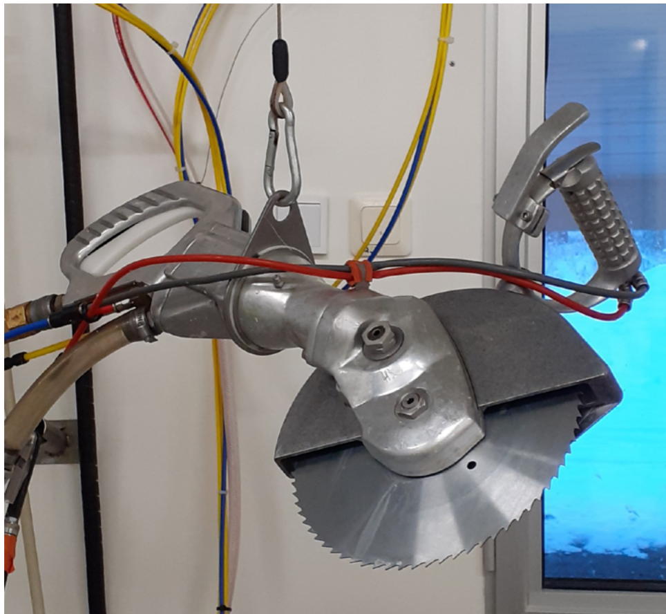
Kuva 1. Tyypillinen teurastamon pienkone (PoSiHIIII -hanke)
