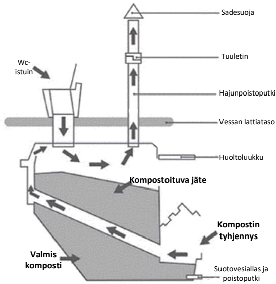
Kuva 13. Kompostikäymälän toiminnan kuvaus. Mustat nuolet kuvaavat käymäläastian ilmankiertoa. (Mukaiillen Hill ym., 2012.)
