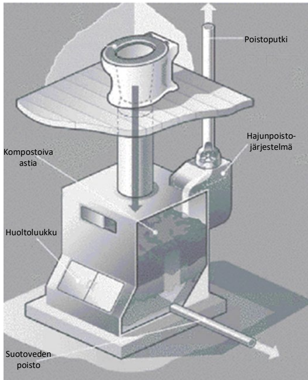
Kuva 12. Vedettömän kompostikäymälän rakenne ja toiminnan kannalta keskeiset osat. (Mukaillen Hill ja Baldwin, 2012.)
