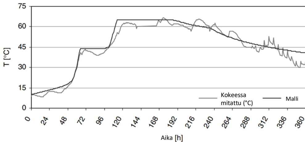
Kuva 5. Kompostin mitattu lämpötilan muutos ajan suhteen. Muutos kuvastaa "kertatäyttöistä" kompostia, jota käytetään perinteisesti mm. puutarha- ja haravointijätteelle. (Mukaillen Sole-Mauri, ym. 2007, 3284.)
