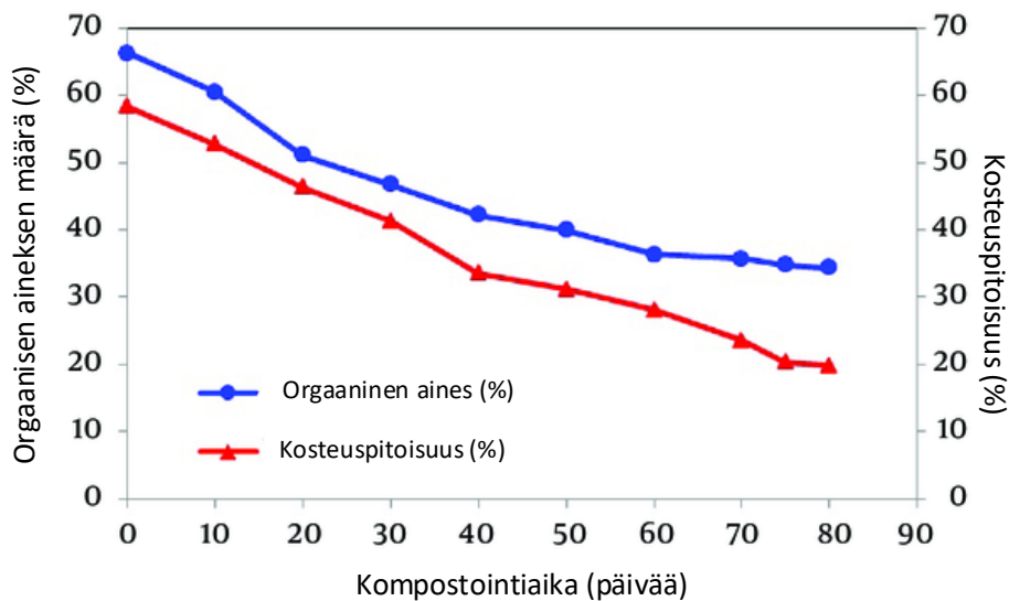
Kuva 8. Kompostin tilavuuden muutosesitys. (Mukaiillen: Bazrafshan, Zarei, Mostafapour, Poormollae, Mahmoodi ja Zazoul, 2016.)
